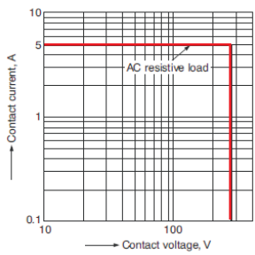
Característica contacto relé
